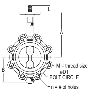
LUG STYLE "LT"
