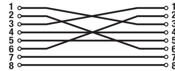
Cableado del cable cruzado
