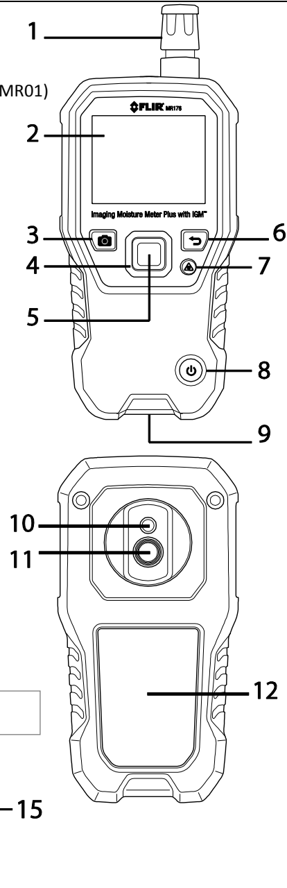
Fig. 4-1 Meter Description
