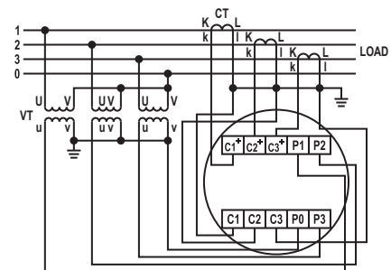
KW 3P4W
