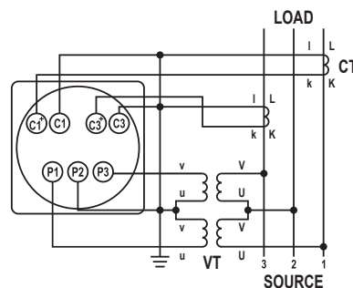
KW 3P3W
