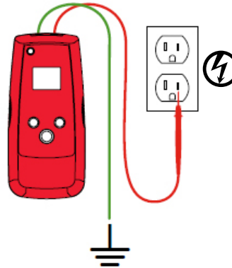
Figura 3.1f Conexión adecuada con conexión a tierra independiente
