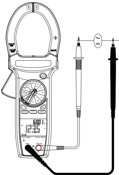
Fig 2. Misure di tensione \ frequenza \ duty cycle
