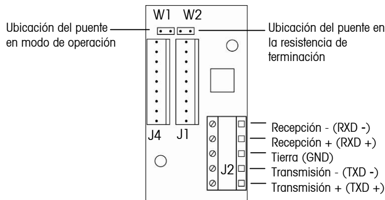
Figura 2.2 Conexiones de la RS485
