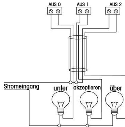
Abbildung 2.4. 6-adrige Relaisverbindung mit externer gemeinsamer Leitung.
