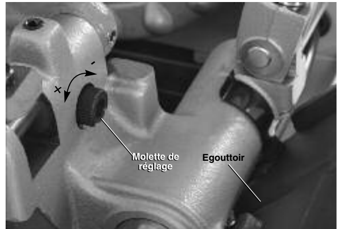
Figure 5 – Réglage du débit d'huile
