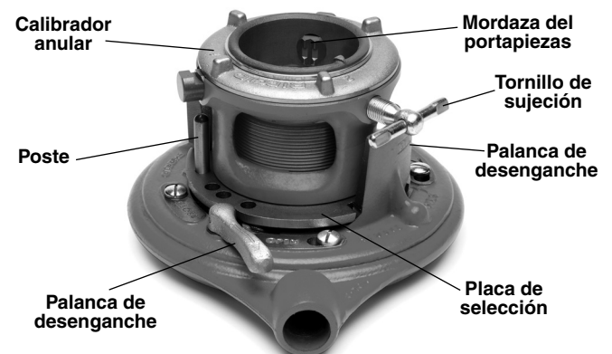
Figura 1 – Roscadora 65R-C
