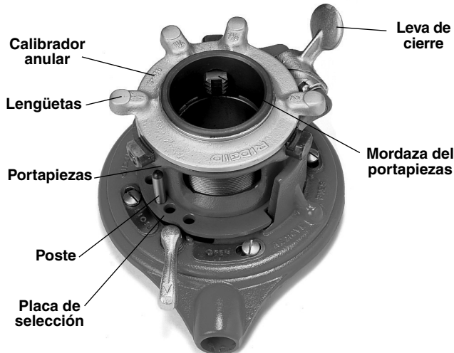
Figura 2 – Roscadora 65R-TC
