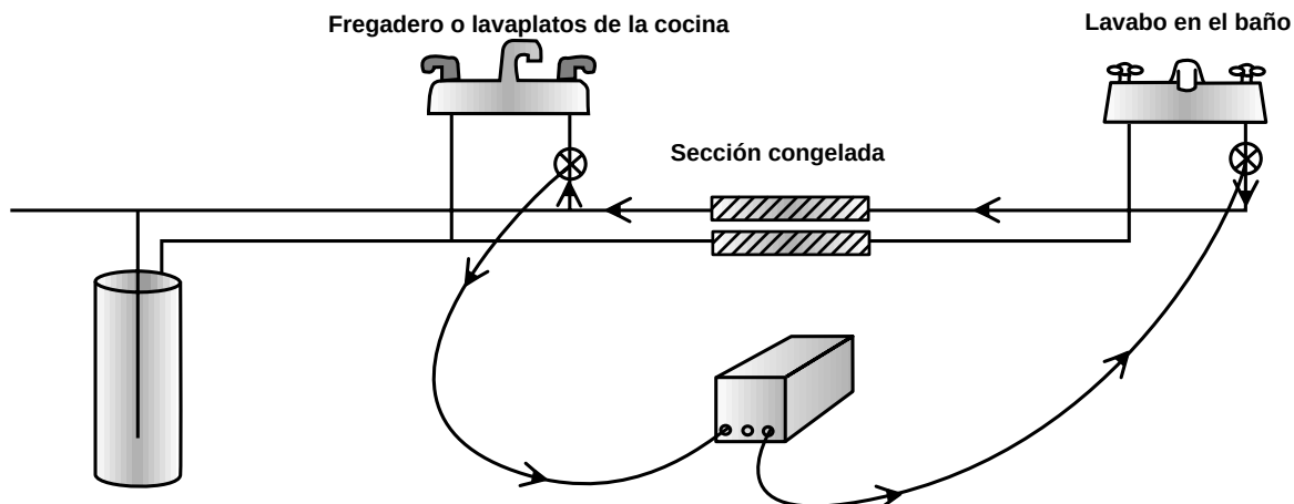
Figure 4 – Descongelación de tuberías domiciliarias de agua potable
