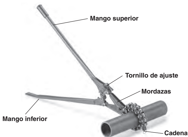
Figura 6 – Cortatubos de desagües cloacales N° 276
