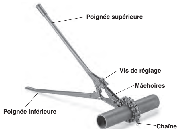
Figure 6 – Coupe-tubes à chaîne n° 276
