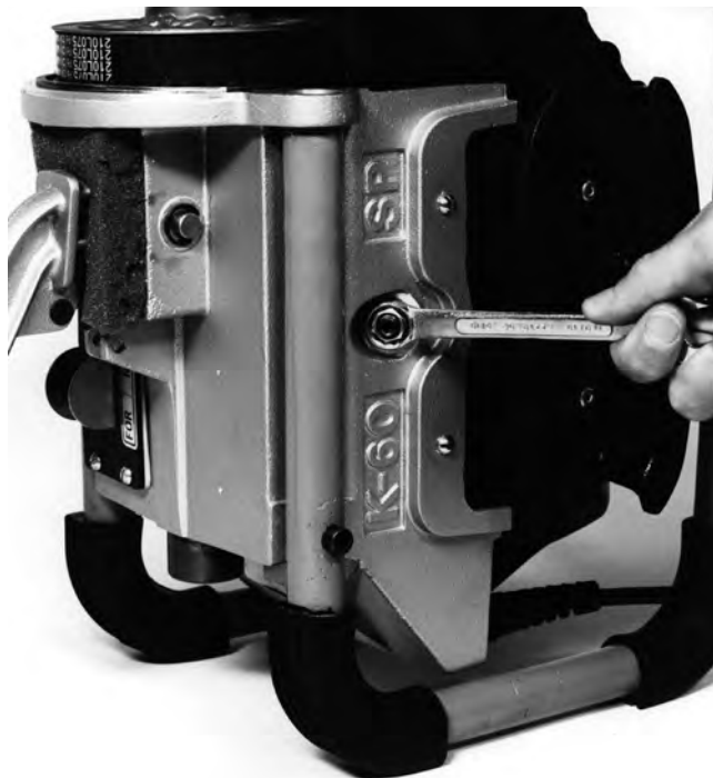
Figure 13 – Desserrez l'écrou de blocage
