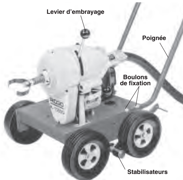
Figure 1 – Dégorgeoir K-1500G
