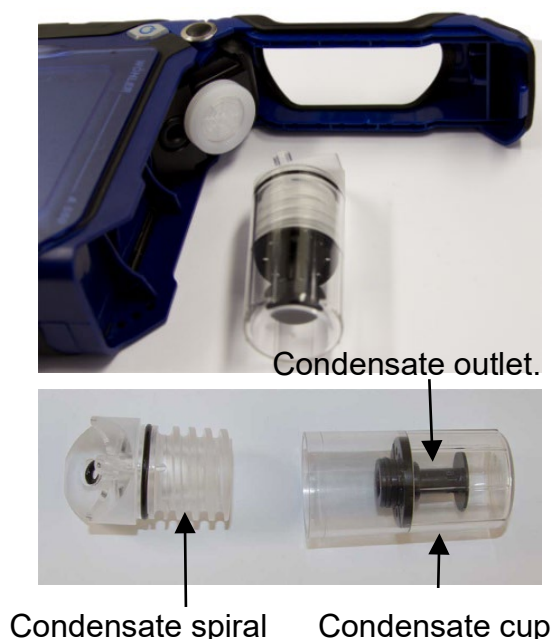
Fig. 68: Condensate trap
