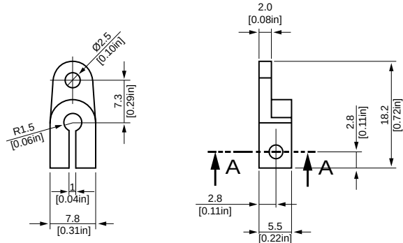
Optional Lever (AX7)
