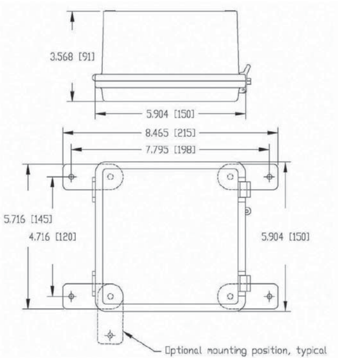
Figure 2 - Dimensions des boîtiers en plastique
