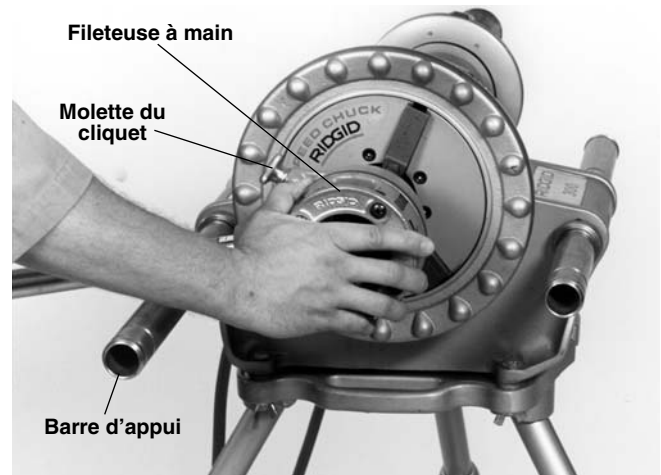
Figure 7 – Enfilage de la fileteuse à main sur le tuyau afin d'engager les filières
