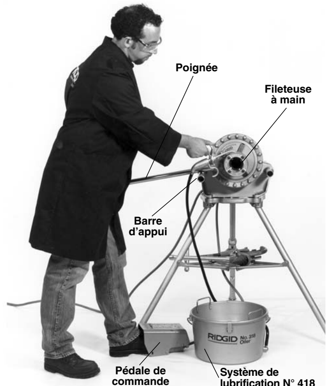
Figure 8 – Filetage à l'aide d'une fileteuse à main
